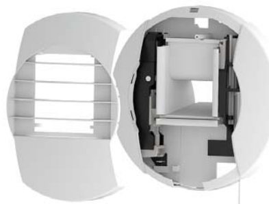
Figure 33 – Bouche d'extraction hygroréglable temporisée SdB/WC communs
